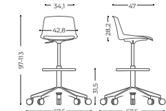
Draughtman chair Banqueta - Elevación gas
